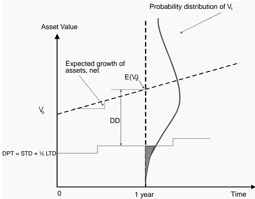
Fig. 16. Distance-to-Default (DD).
